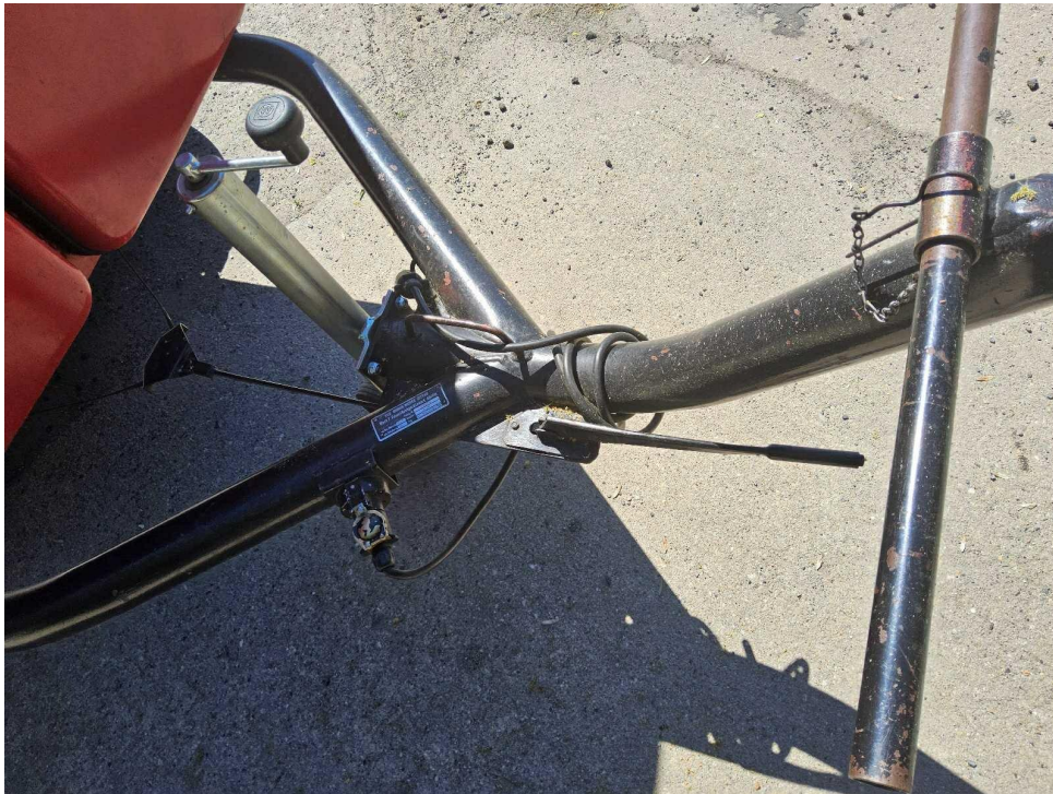
Bild 11 : Feststellbremse
