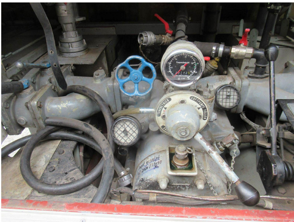
Bild 14 : Löschwasserpumpe
