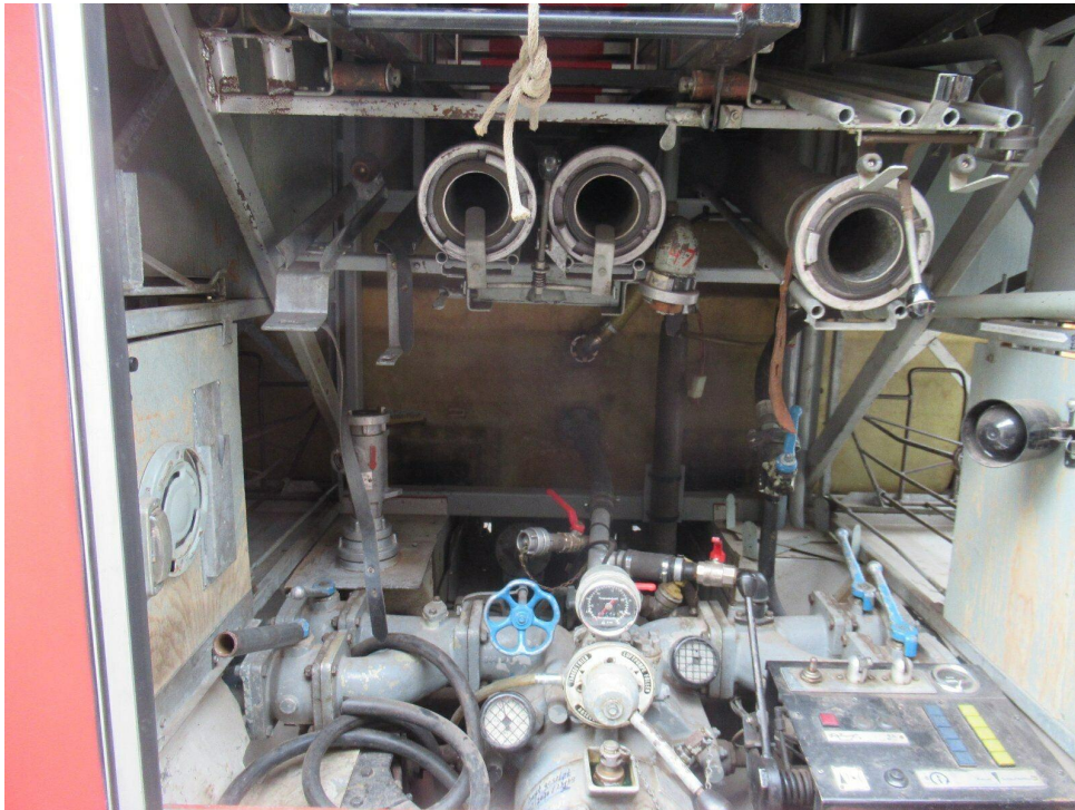
Bild 13 : Technik Heckklappe Löschpumpe mit Zubehör
