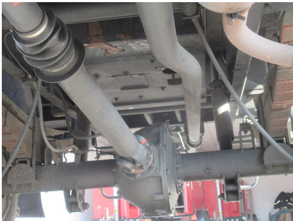
Bild 16 : Differential Hinterachse
